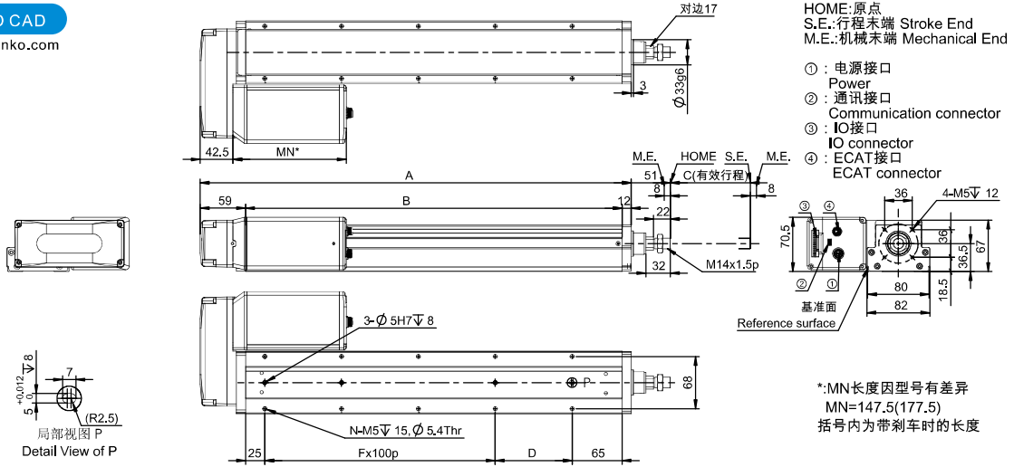
尺寸图代号说明 · 质量 Dimensions, Mass
