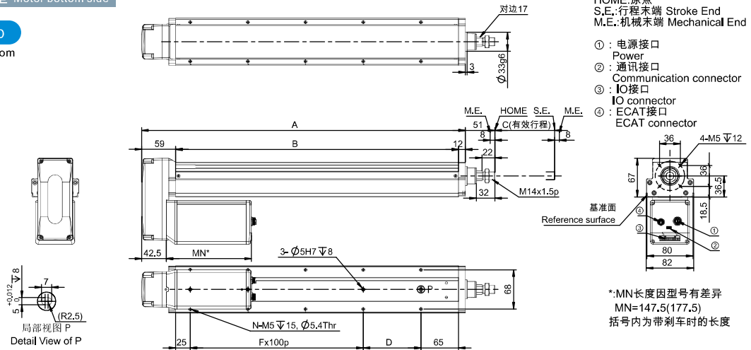
尺寸图代号说明 · 质量 Dimensions, Mass
